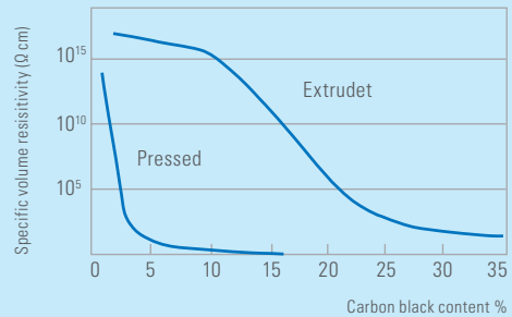
单位容积电阻与碳黑含量相关的容积电阻
